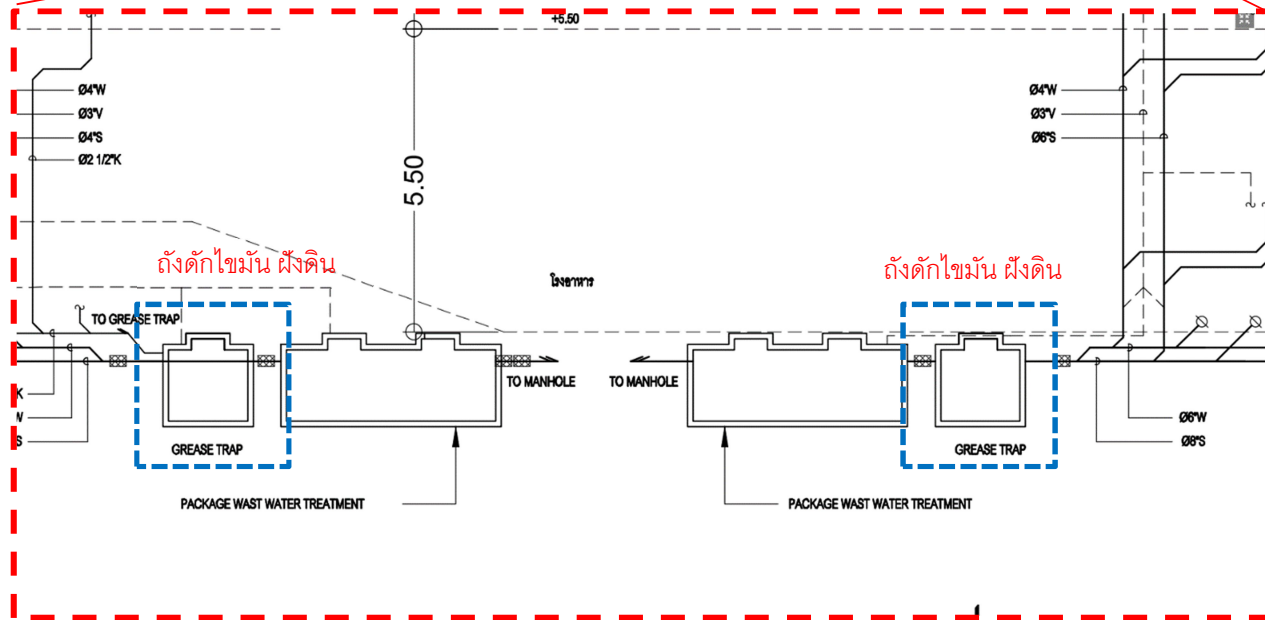
ผังแสดงตำแหน่ง ถังดักไขมัน ชนิดฝังดิน ประจำอาคาร 36
